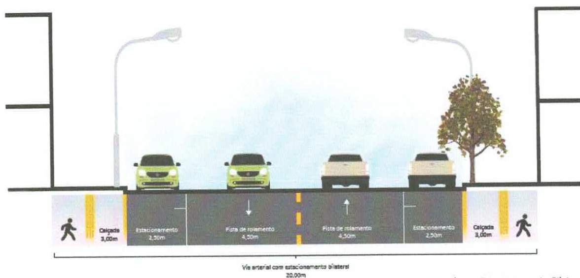
Via Arterial com Estacionamento Bilateral Escala 1/125
