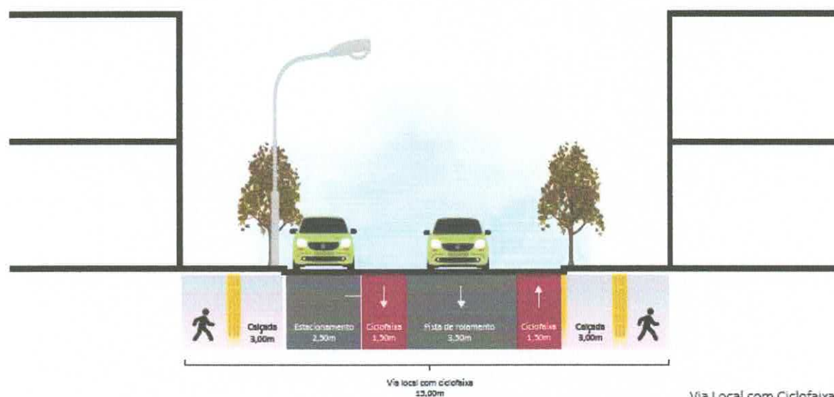
Via Local com Ciclofaixa Escala 1/125
