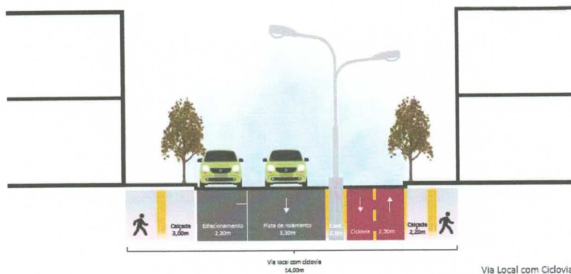
Via Local com Ciclovia Escala 1/125
