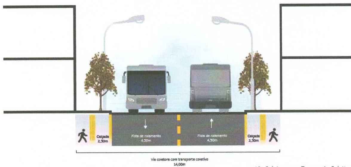
Via Coletora com Transporte Coletivo Escala 1/125
