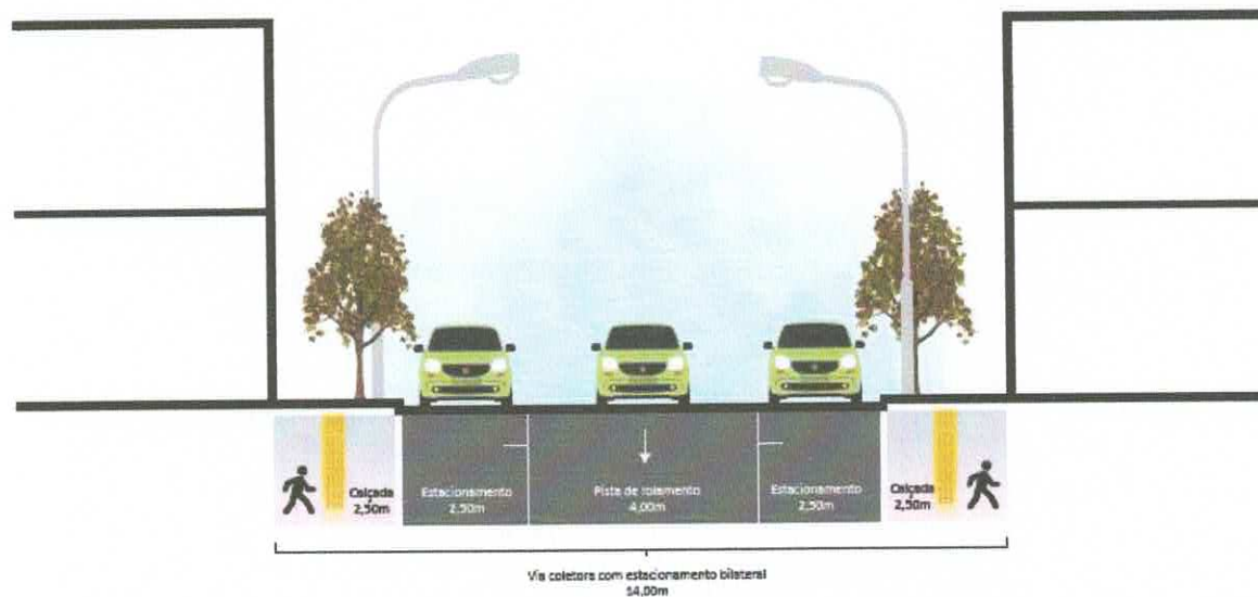
Via Coletora com Estacionamento Bilateral Escala 1/125
